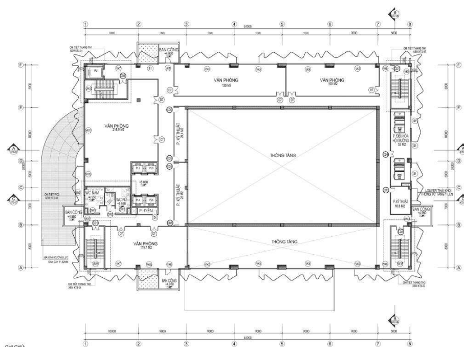
MẶT BẰNG TẦNG LỬNG 1473,8 M 2
