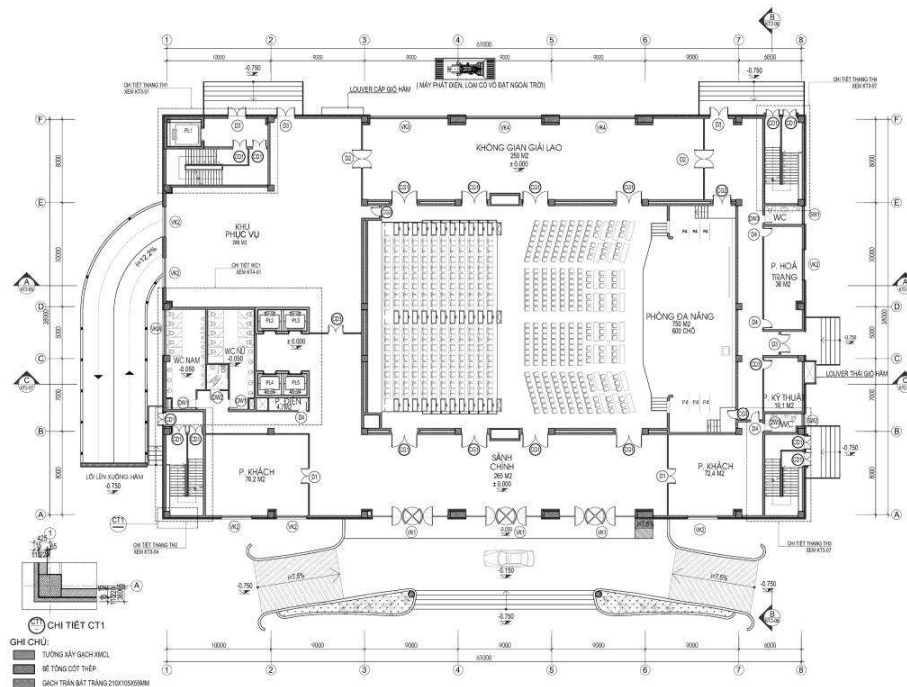
MẶT BẰNG TẦNG 1 2377,7 M 2
